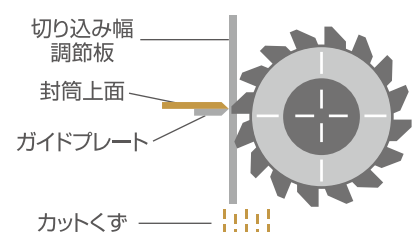
ミリングカットイメージ図
